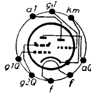
Sockelschaltungsdiagramm
